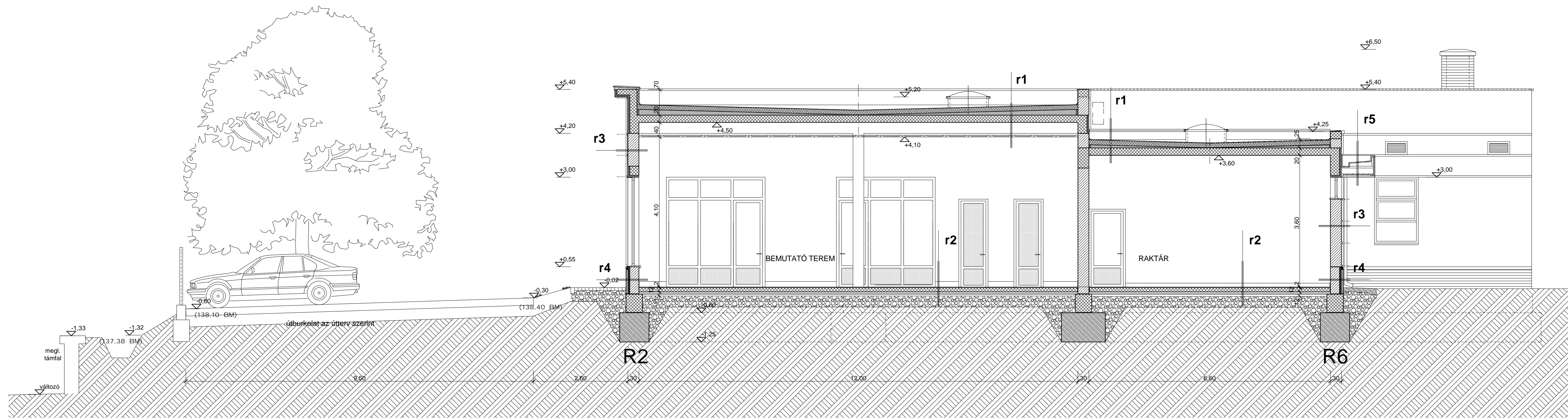
A-A KERESZTMETSZET
