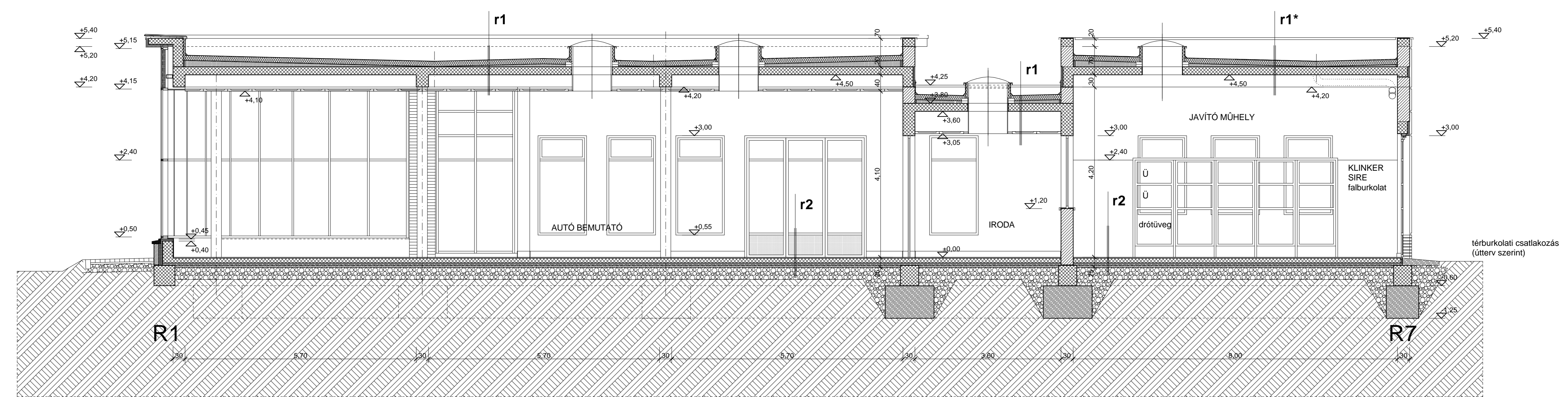
B-B HOSSZMETSZET
